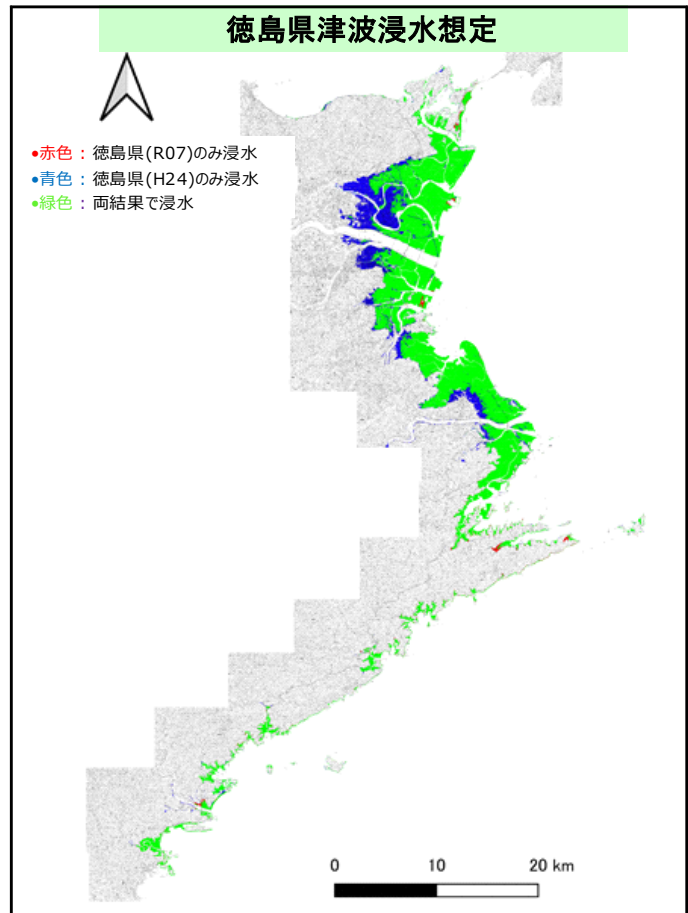
図：津波浸水想定（比較）
