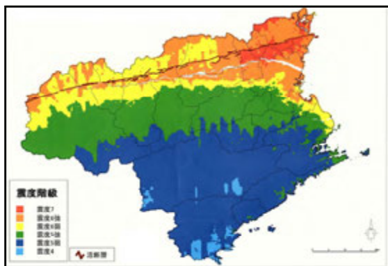
図：震度分布
